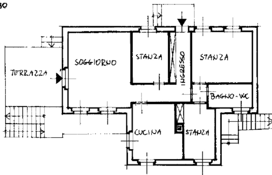
PIANTA PIANO SEMINTERRATO H=2.30
