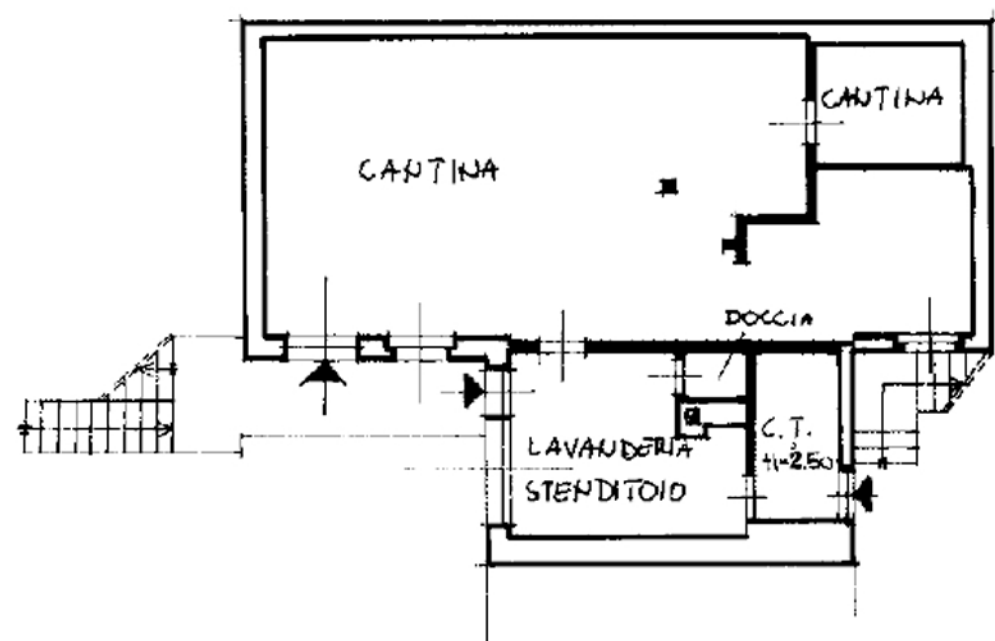
PIANTA PIANO SEMINTERRATO H=2.30
