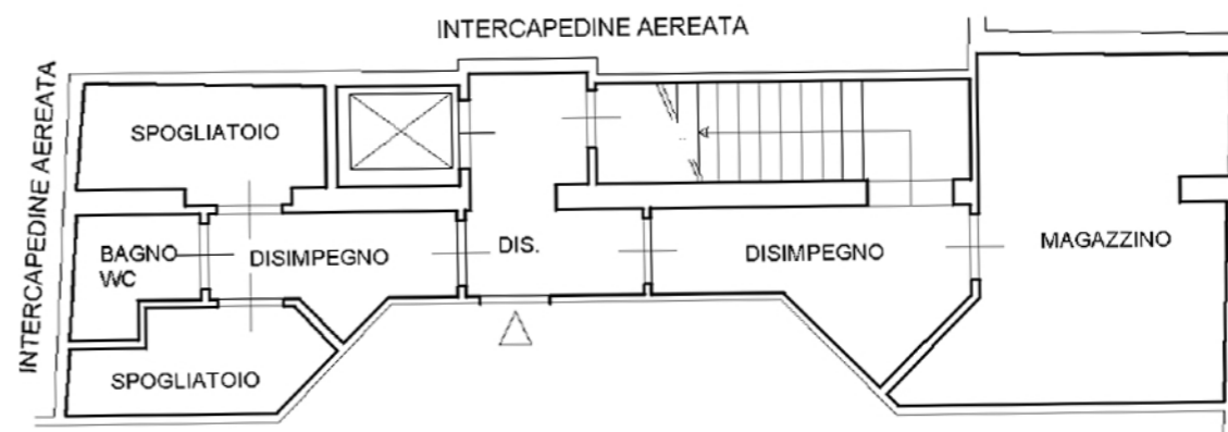
PIANO PRIMO SOTTOSTRADA H=2.40
