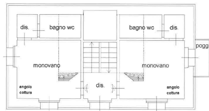
Primo piano h.4.30
